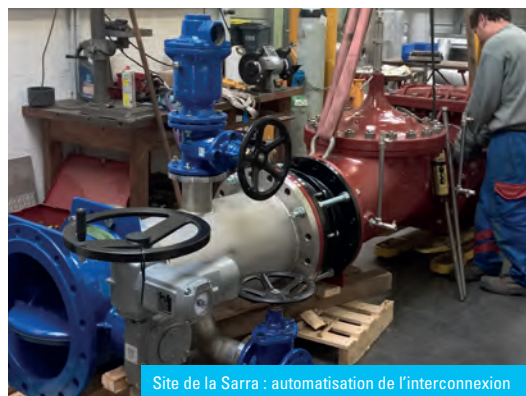
Site de la Sarra : automatisation de l'interconnexion
